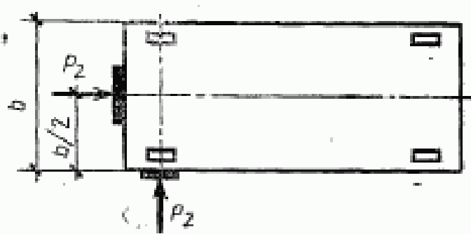
b — ширина изделия Черт. 9
