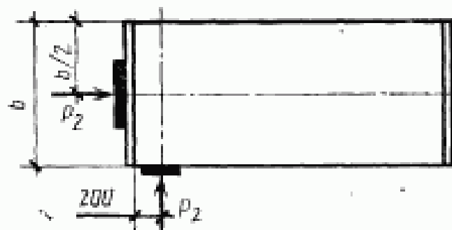
b — ширина изделия Черт. 10
