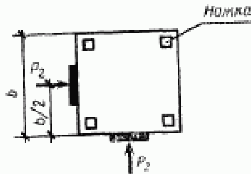
b — ширина изделия Черт. 8
