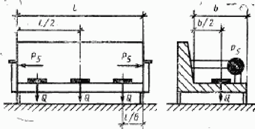
l — ширина посадочных мест; b — глубина посадочного места
